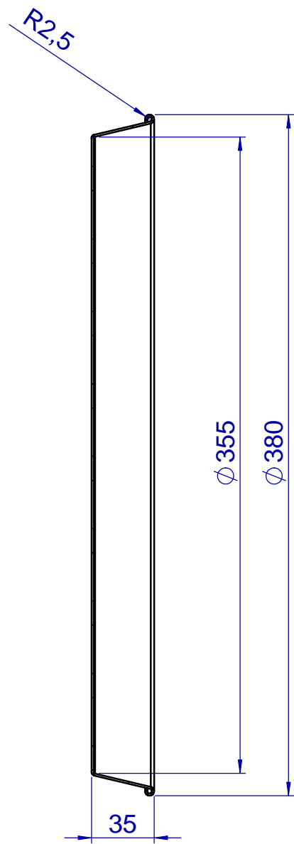
SEZIONE A-A
